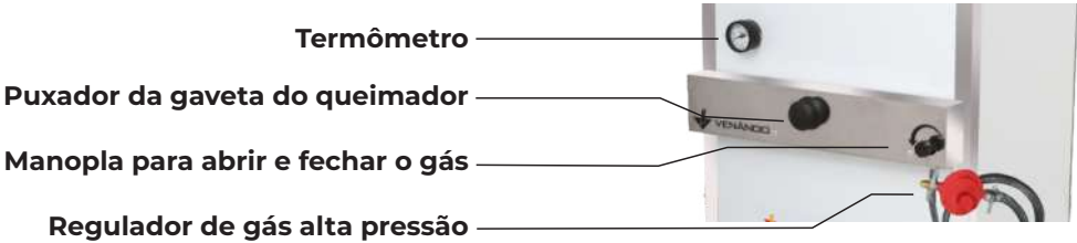
Regulador, com mangueira, que será conectado ao botijão ou a central de gás.
