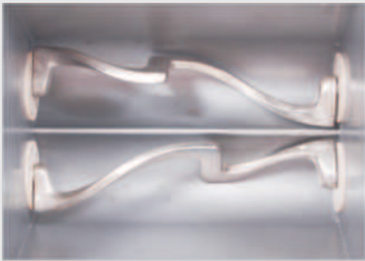
Batedores em ferro fundido nodular (estanhado)
